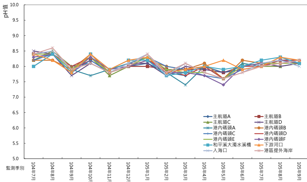
圖 2.12-1 底泥重金屬 pH 監測結果
