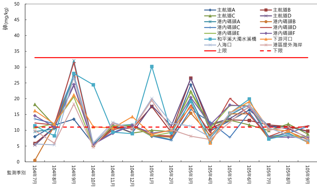
圖 2.12-2 底泥重金屬砷監測結果
