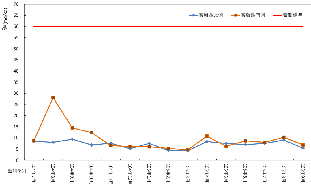
圖 2.13-2 土壤重金屬砷監測結果
