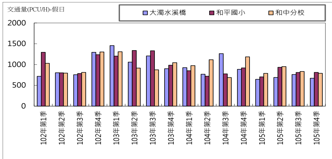
圖 2.7-1 營運後歷次交通流量比較分析圖(假日)
