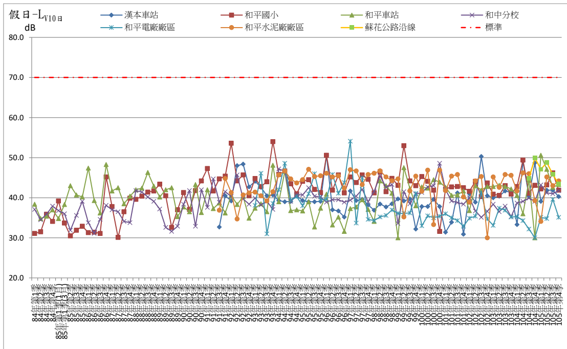
圖 2.2-4 歷年假日振動( L_{v10日} )與歷次監測結果比較圖
