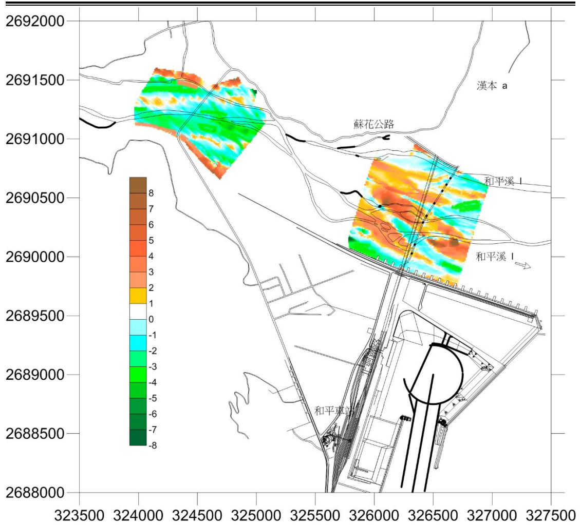
圖 2.9-1 和平地區鐵公路橋基地形監測侵淤變化圖 (86.12~105.11)
