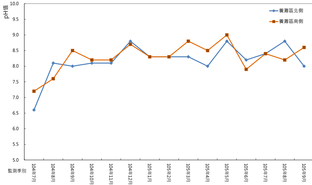
圖 2.13-1 土壤重金屬 pH 監測結果
