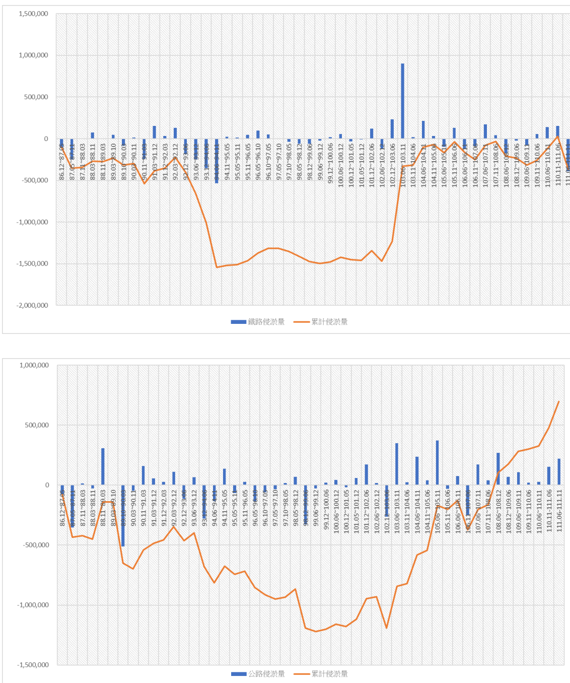
圖 2.9-2 鐵公路橋基侵淤量累積變化圖
