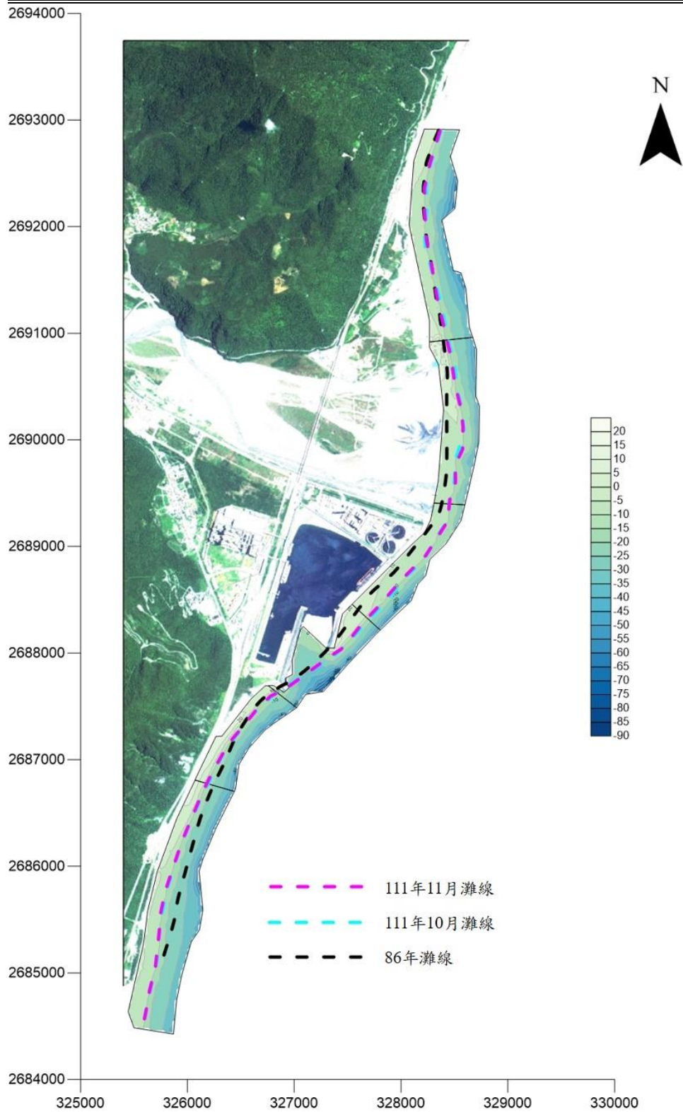
圖 2.8-2 和平地區海岸地形監測侵淤及灘線變化圖
